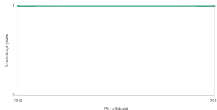
Кількість цитувань за роками
