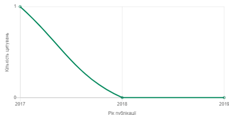
Кількість цитувань за роками
