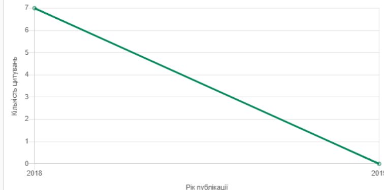
Кількість цитувань за роками
