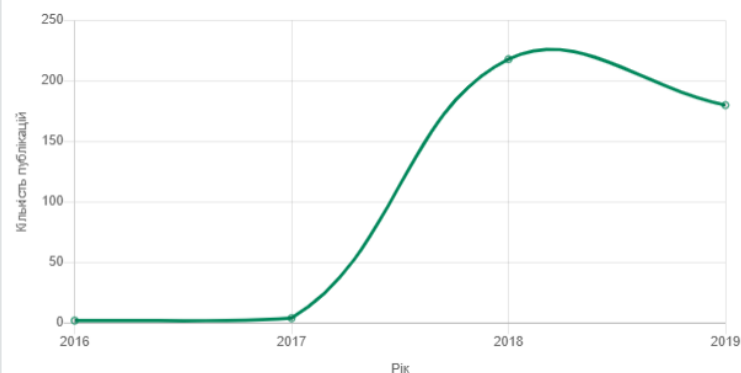
Кількість публікацій за роками
