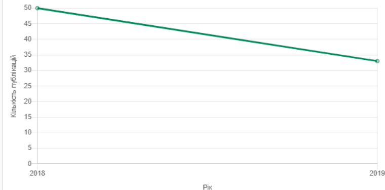
Кількість публікацій за роками
